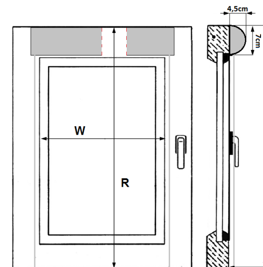
Miejsce montażu kasety i prowadnic
